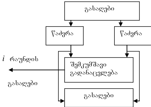
სურ.3.3. რაუნდის გასაღების გამომუშავების სქემა
