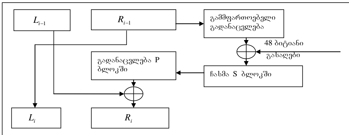
სურ. 3.4 DES-ის ერთი რაუნდის სქემა
