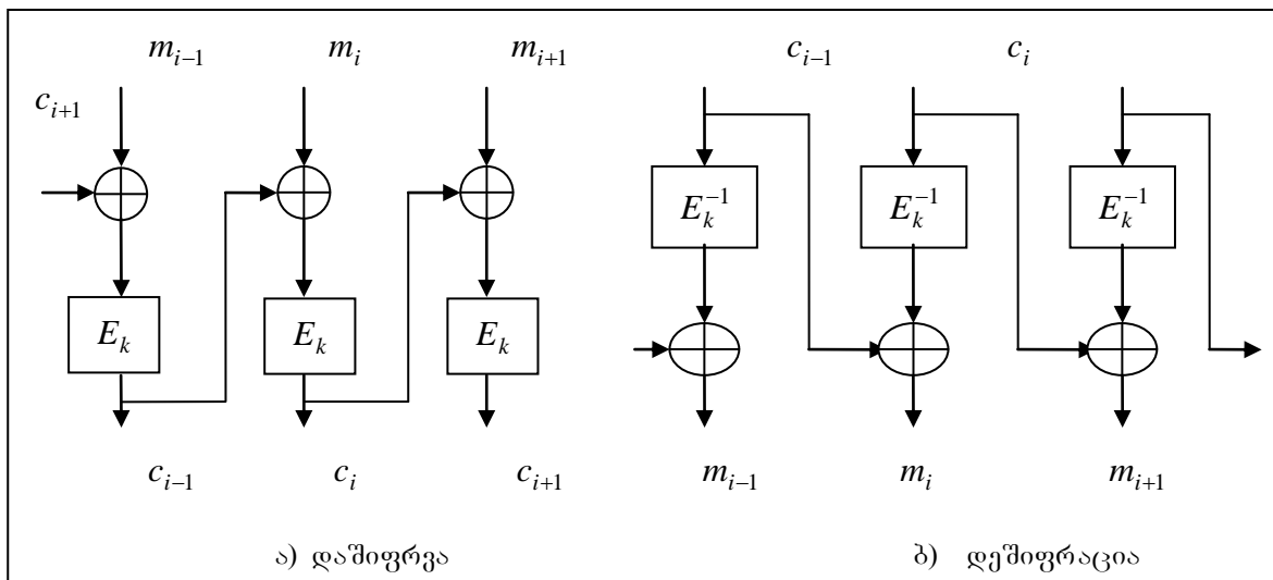
სურ. 4.6 CBC რეჟიმი.
